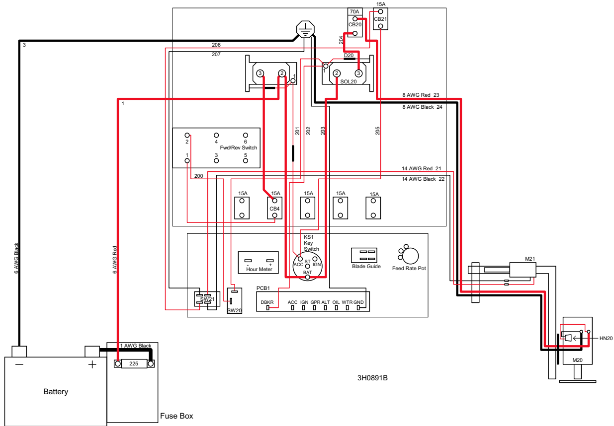
FIG. 5-5
