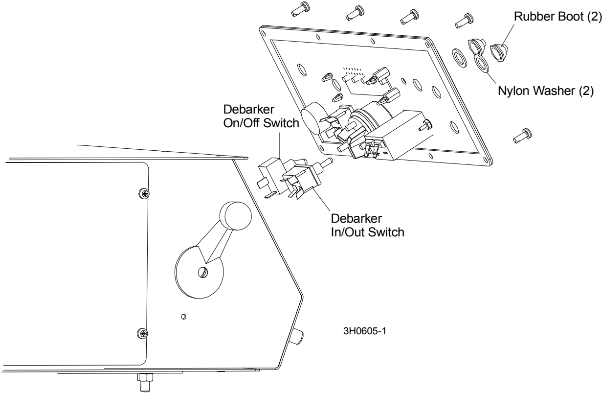
FIG. 2-15
