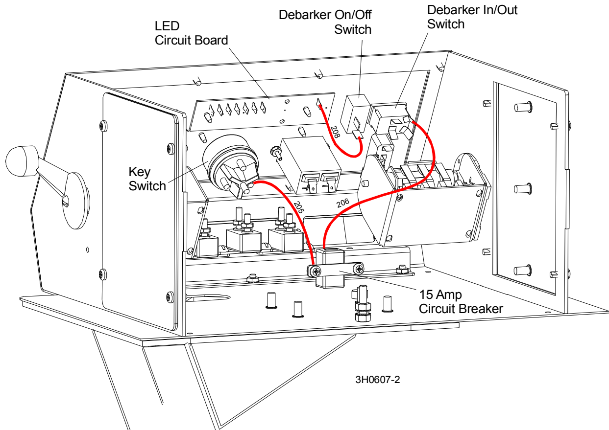
FIG. 2-16
