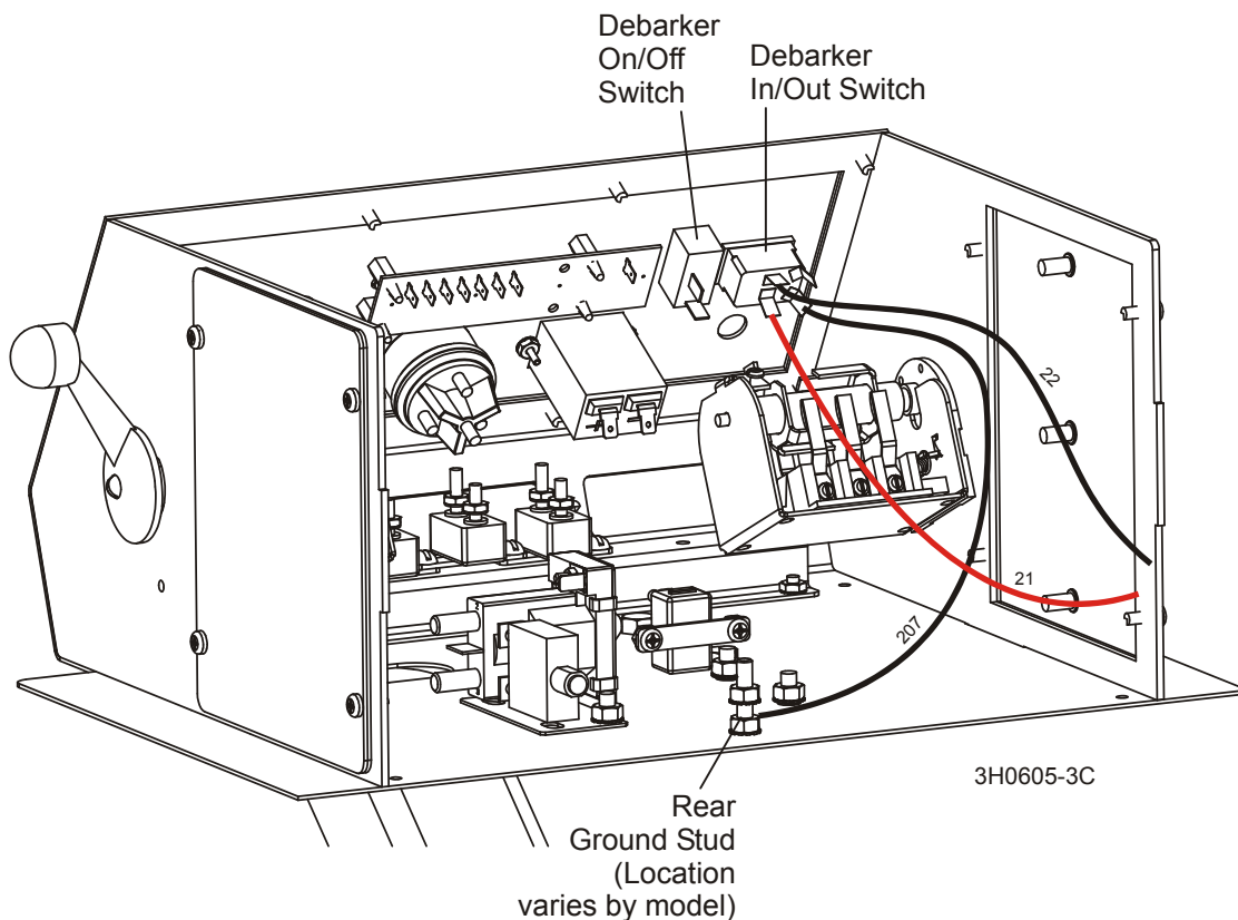
FIG. 2-12
