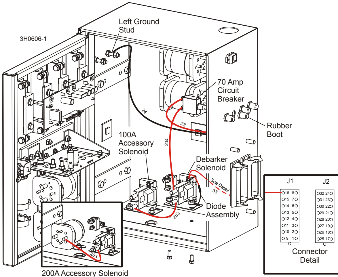
FIG. 2-13
