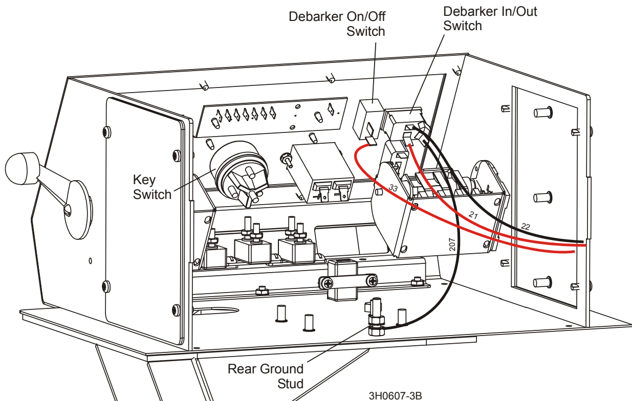
FIG. 2-18
