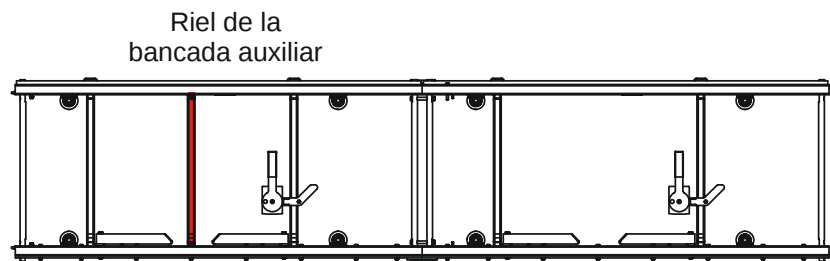
Vista Superior - El aserradero estándar con dos bancadas
