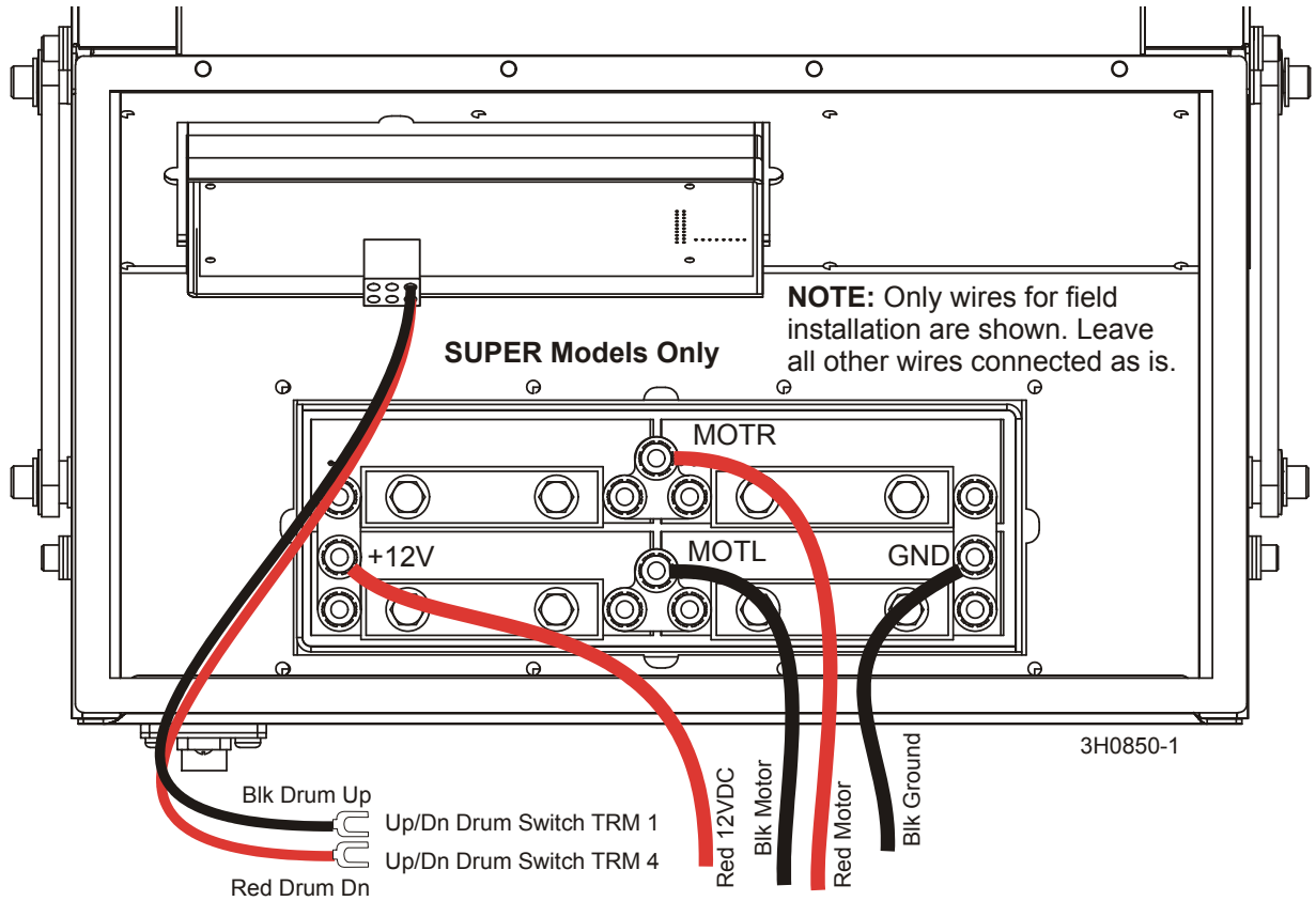
FIG. 1-21 SCIERIES DE LA GAMME SUPER UNIQUEMENT
