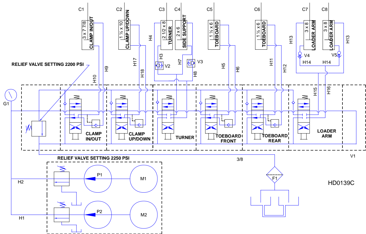
FIG. 8-1 DIAGRAMA HIDRÁULICO.
