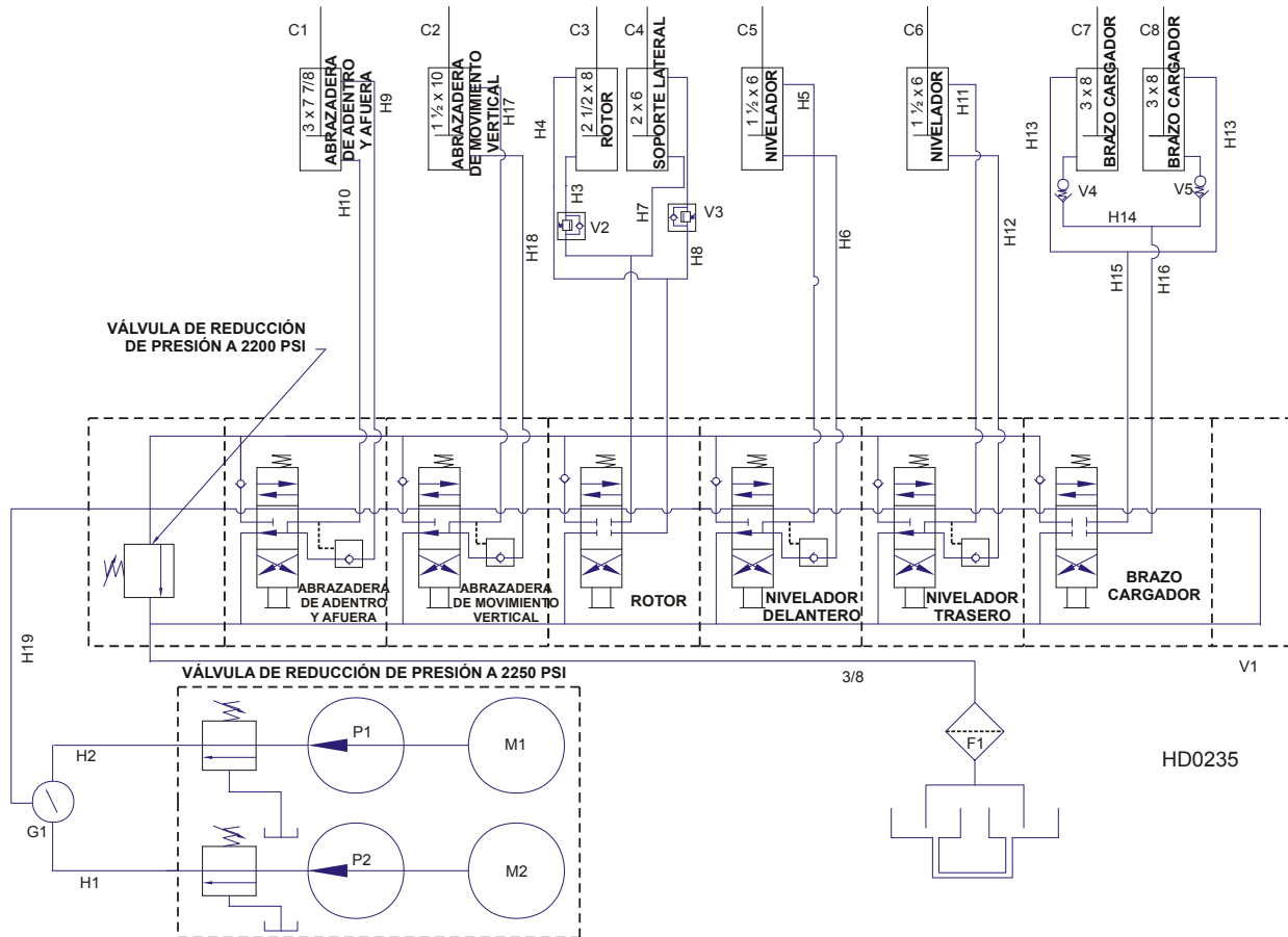
FIG. 8-1 DIAGRAMA HIDRÁULICO.
