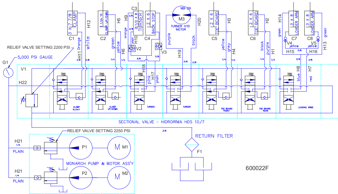
FIG. 8-1 SCHÉMA HYDRAULIQUE
