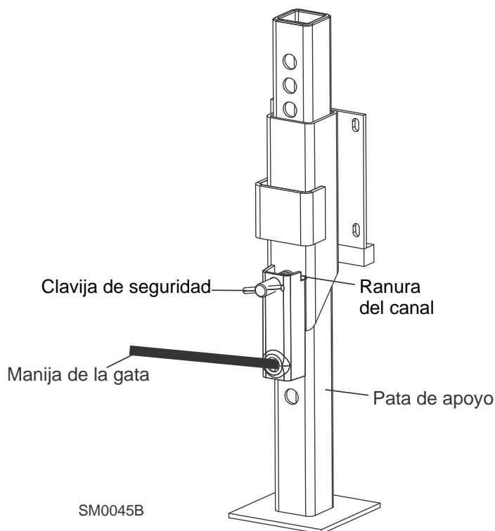
FIGURA 3-10. AJUSTE DEL BALANCÍN.
