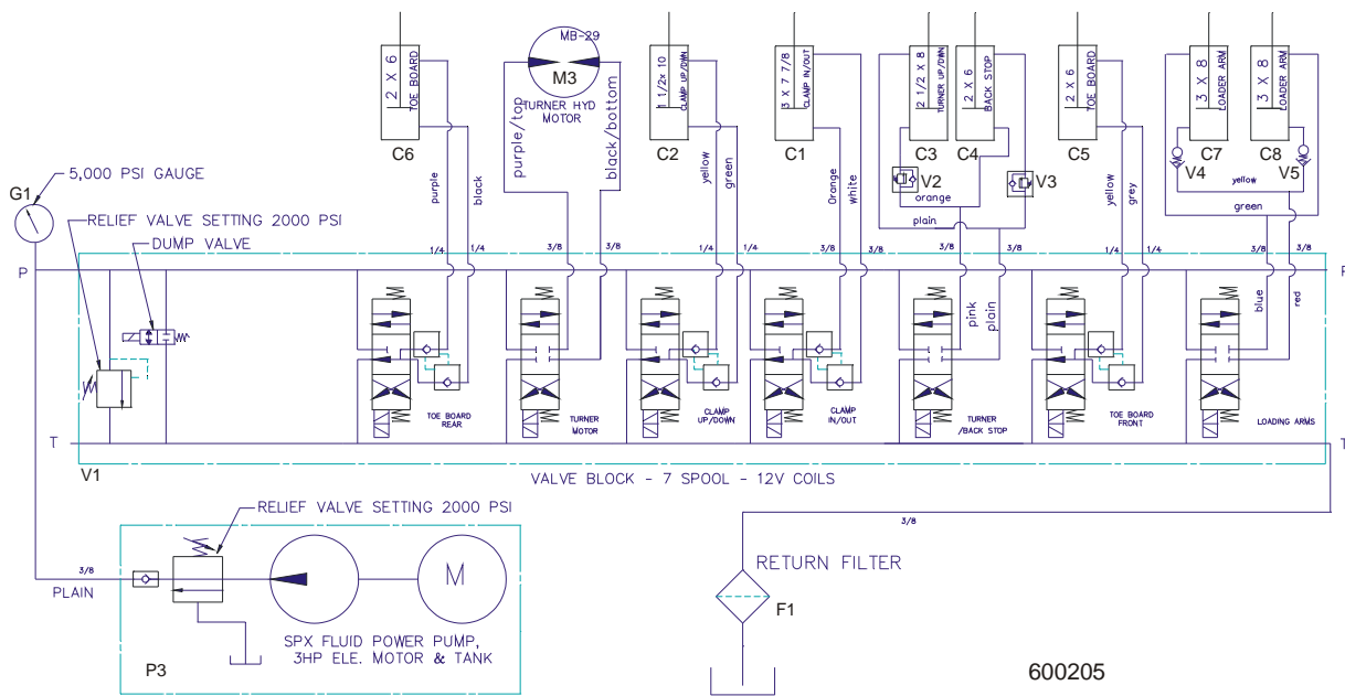
FIG. 8-2 DIAGRAMA HIDRÁULICO (MODELOS REMOTOS DE CA)
