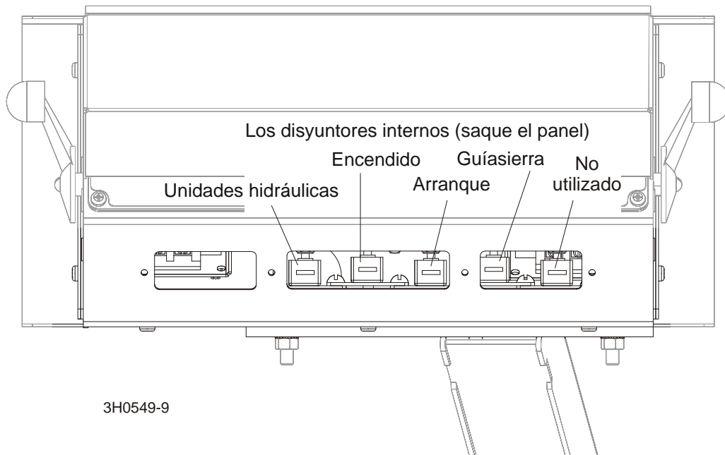
FIG. 6-3 MODELOS DE CA SOLAMENTE
