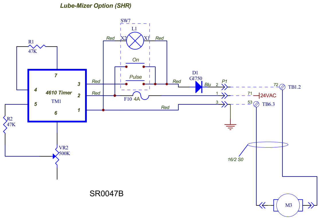
FIG. 1-14 SYMBOL DIAGRAM (LUBE-MIZER)
