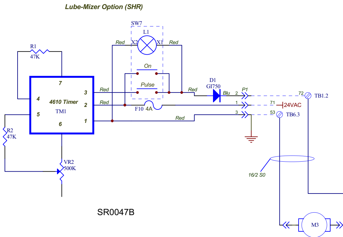
FIG. 1-7 SYMBOL DIAGRAM (LUBE-MIZER)
